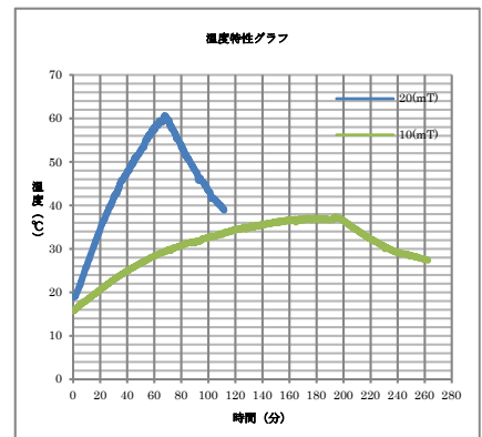
温度特性
