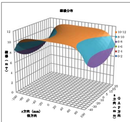
分布精度
