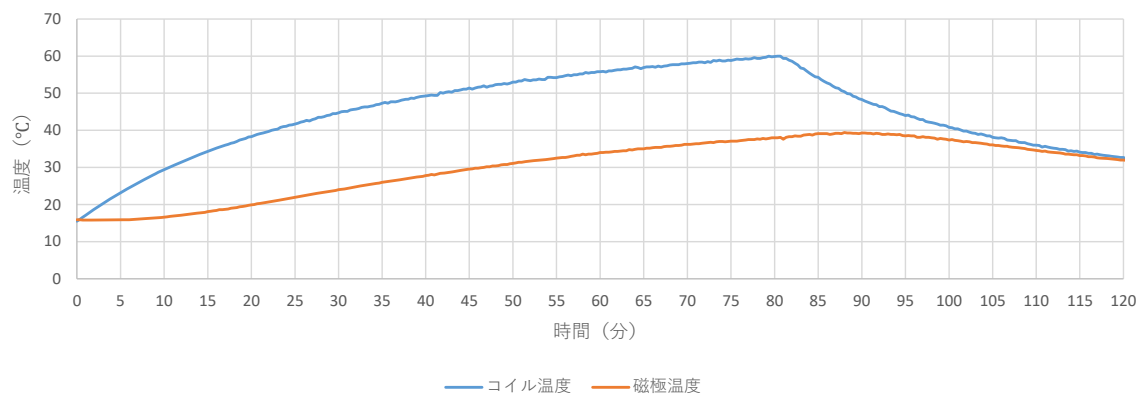
3 A 連続運転試験
